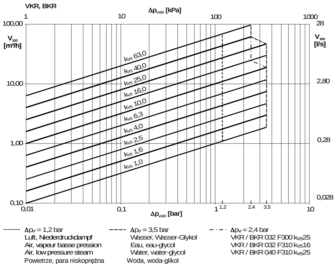
Wykres natężenia przepływu
