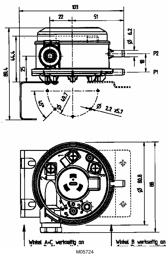
Rysunek wymiarowy
