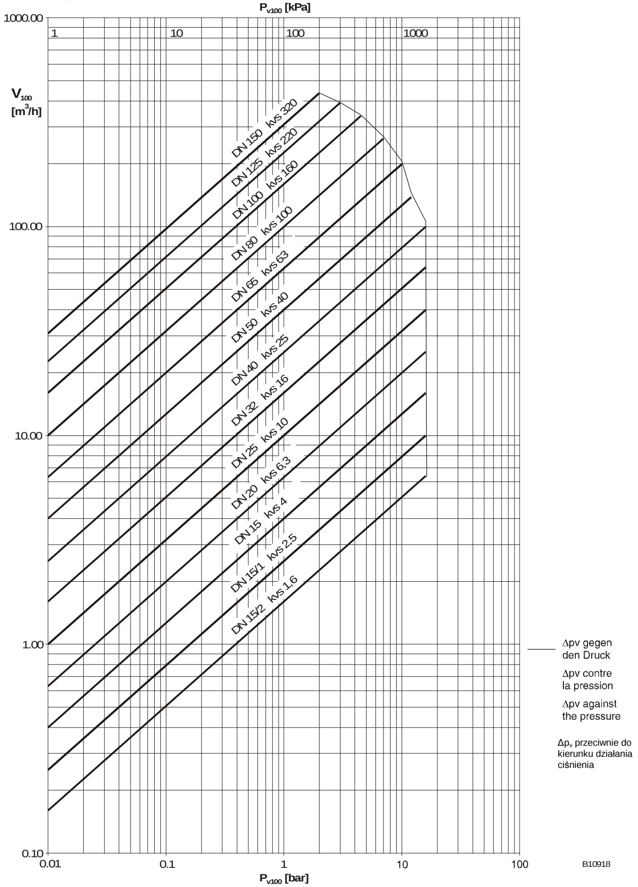
Wykres natężenia przepływu (zawór BUS)
